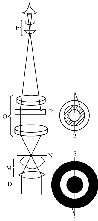
图 2-1 相差显微镜光路图解
