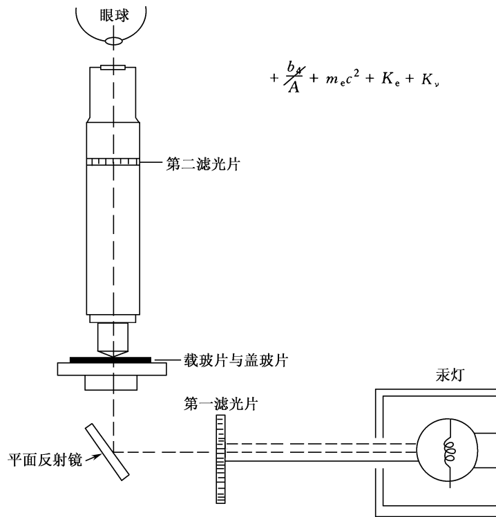
图 2-2 透射式荧光显微镜图解
