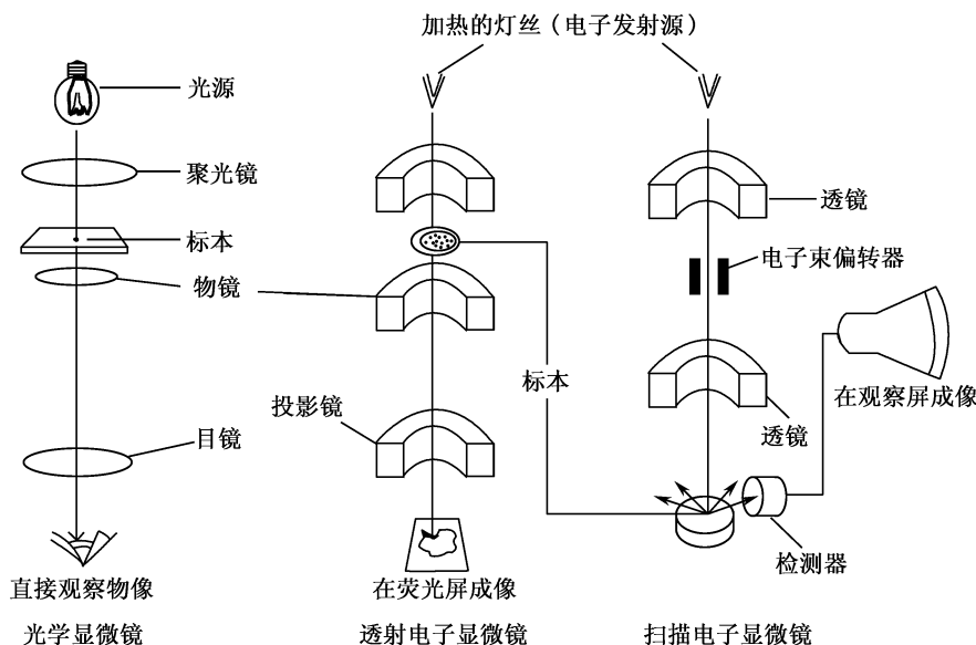
图 2-4 光镜、透射电镜和扫描电镜的主要特征示意图
