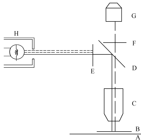
图 2-3 落射式荧光显微镜图解
