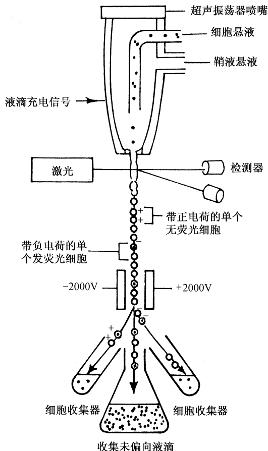
图 2-6 流式细胞仪原理图解
