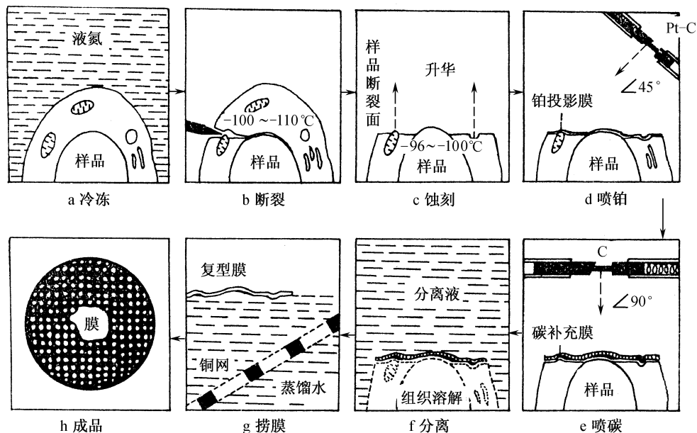
图 2-5 冰冻蚀刻复型电镜技术操作步骤示意图
