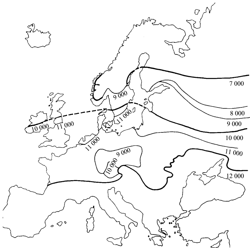
图 2.3 反映栎属 ( Quercus ) 晚冰期以来在欧洲迁移过程的孢粉等时线图 图中的数字为年代 (aBP) (引自 Gliemerth, 1995)
