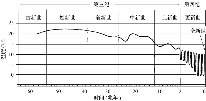
图 1.1 第三纪和第四纪地球温度的变化过程示意图 (引自 Lang, 1994)
