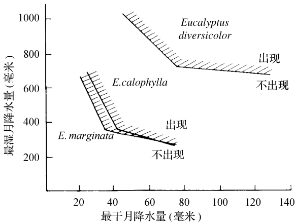
图 2.1 澳大利亚三种桉树的生长受降水条件的限制作用 (引自 Churchill, 1968)
