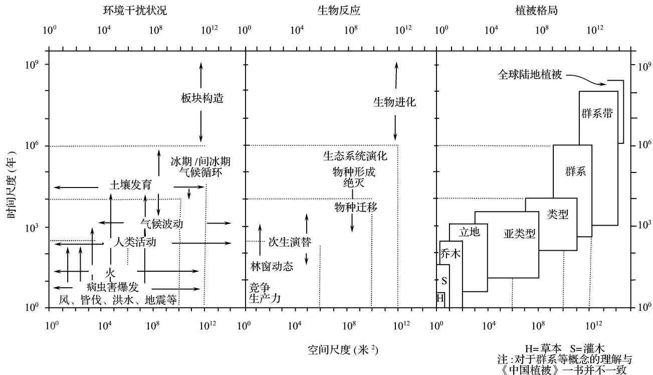
图 1.2 不同时空尺度下的环境干扰与生物反应(引自 Delcourt and Delcourt, 1991)
